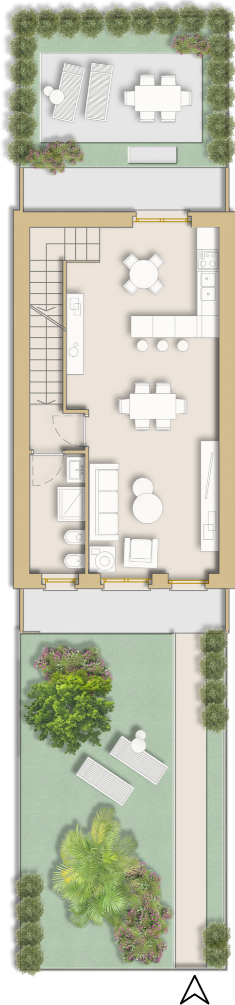
PIANO TERRA CON GIARDINO
